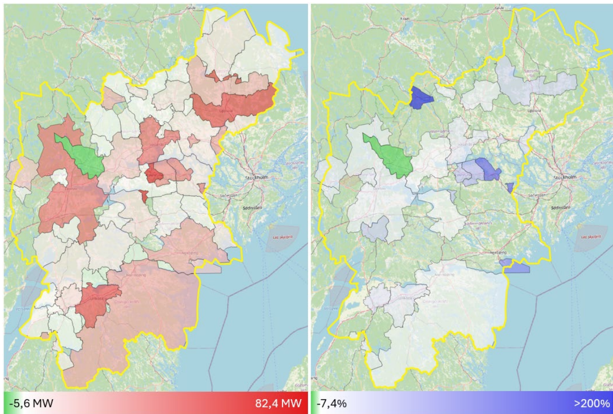
Figur 3 - Tillkommande behov av överföringskapacitet i lokalnäten för förbrukarbehov 2034 per delområde. Kartan till vänster redovisar behov av överföringskapacitet och kartan till höger redovisar procentuell förändring jämfört med utgångsvärdet 2024.
